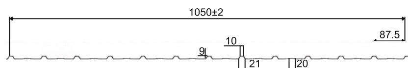
Biên dạng tôn 13 sóng la phong - H9 - khổ 1200
