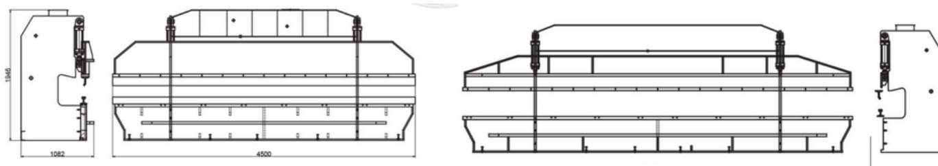
Layout máy chấn thường 4.5m
